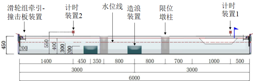
(b) 主视图
