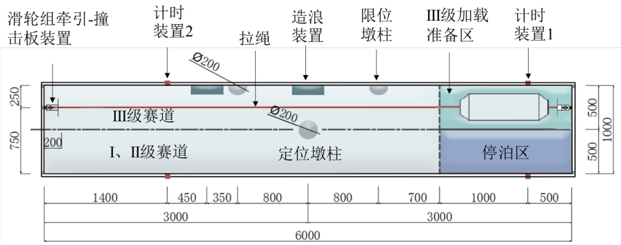
(a) 俯视图
